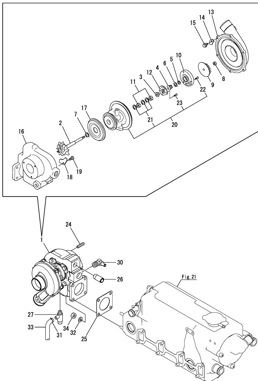
Fig.11. TURBINE(4JH4-TE)
