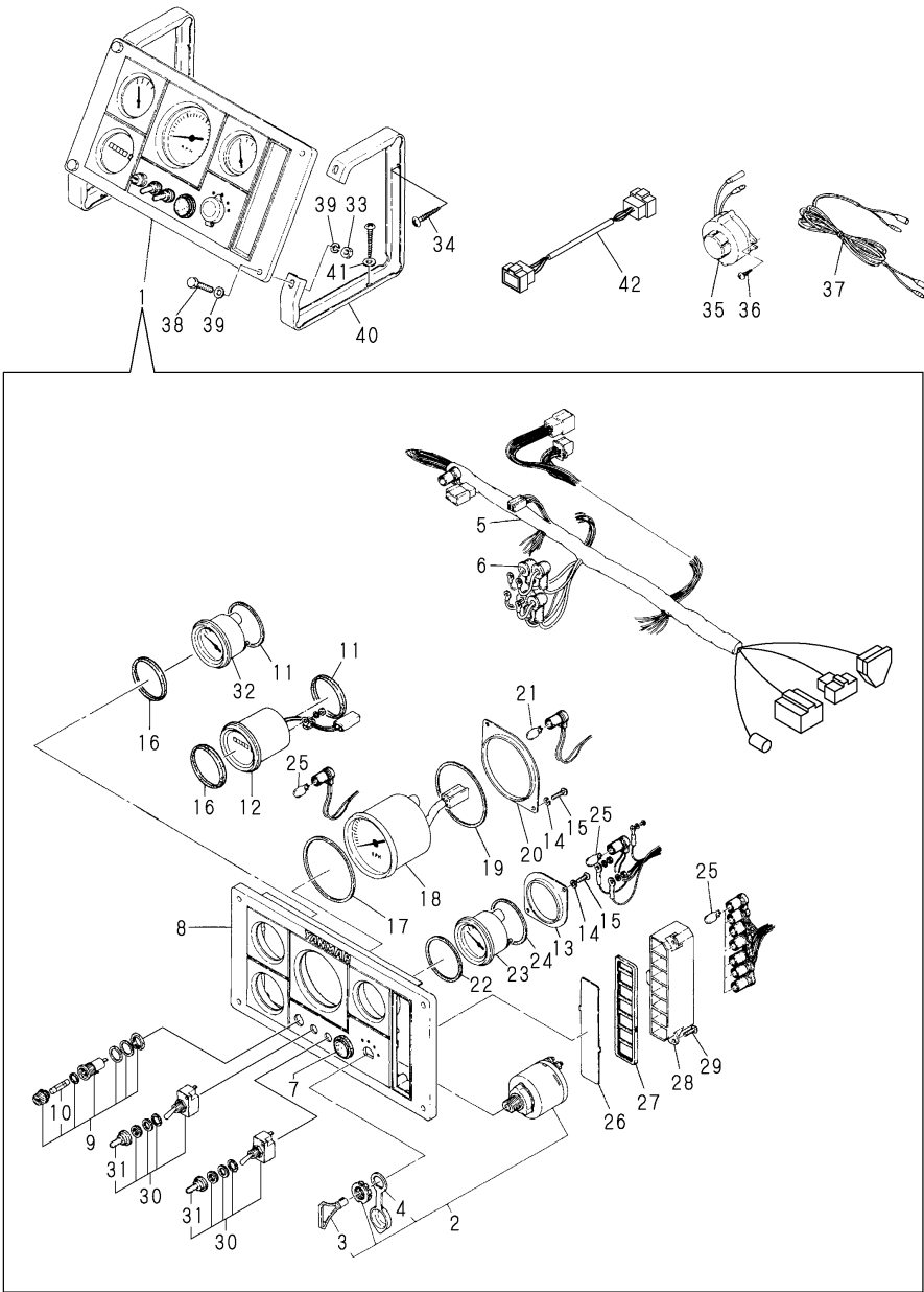
Fig.61. INSTRUMENT PANEL(C:4JH3-TE)
