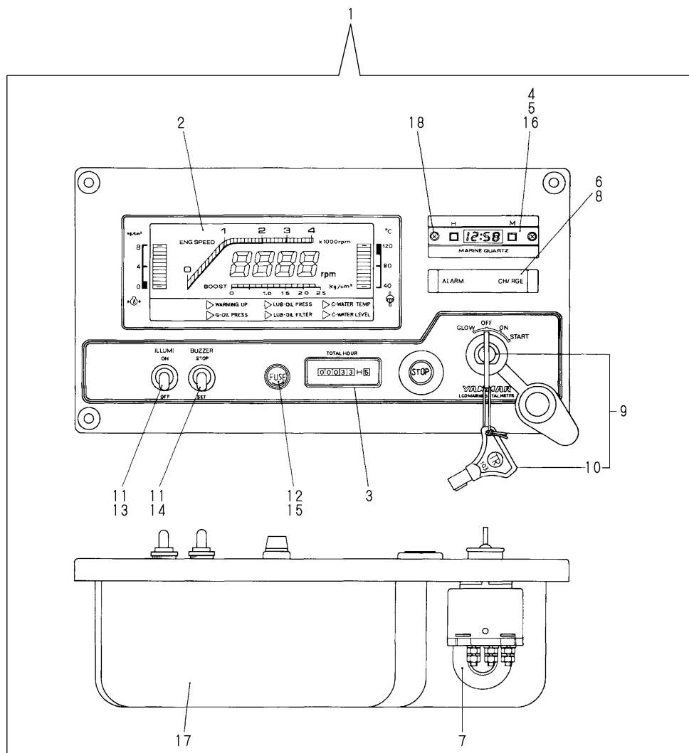
Fig.63. INSTRUMENT PANEL(E:4JH3-TE)
